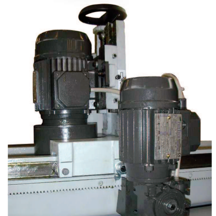
Rack movement of the head. Bewegung des Kopfes mit Zahnstange. Перемещение головки по зубчатой рейке
